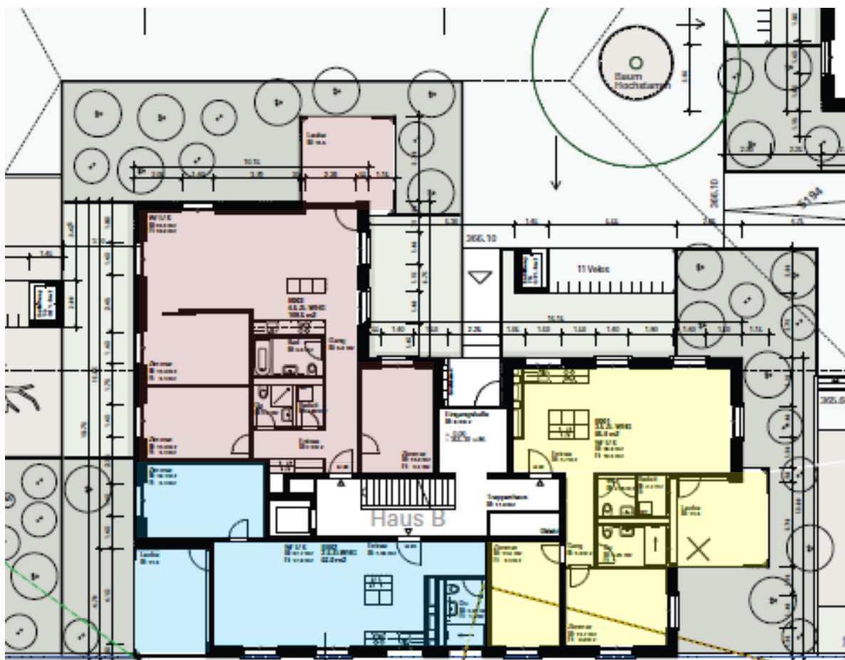
Grundriss Haus B (Beispiel)
