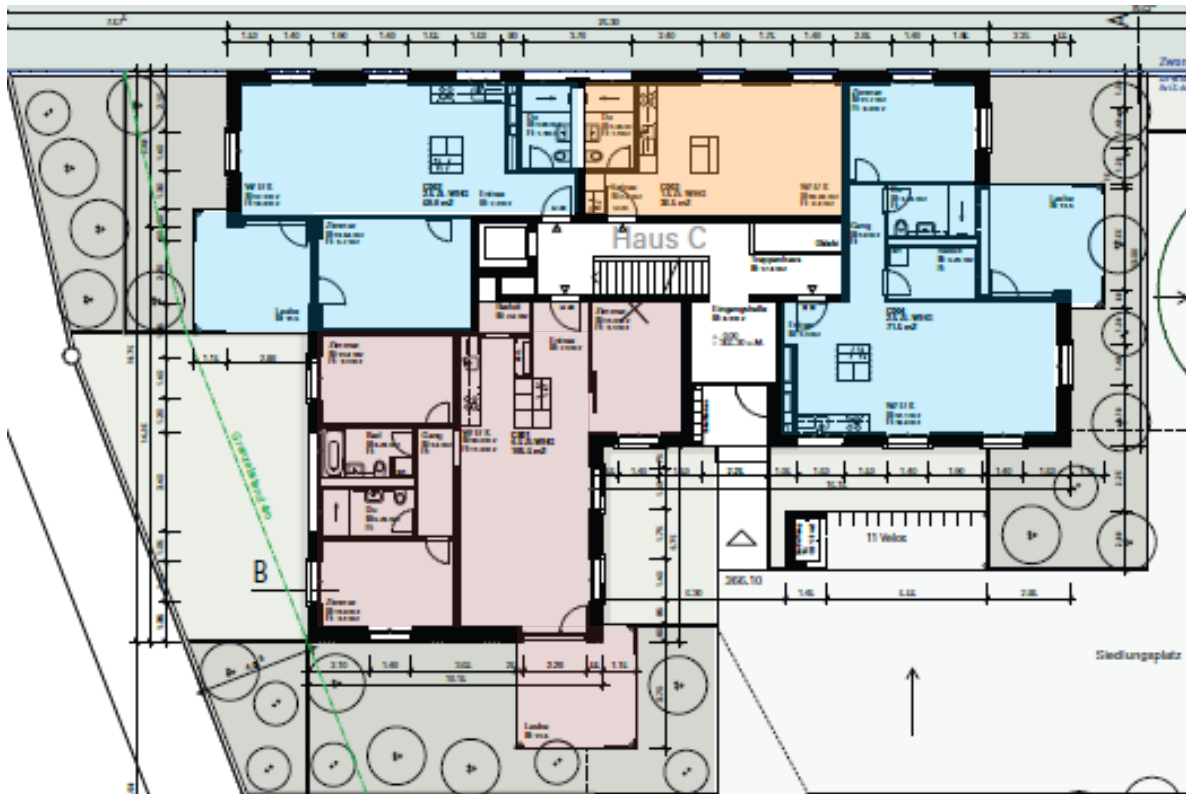
Grundriss Haus C (Beispiel)
