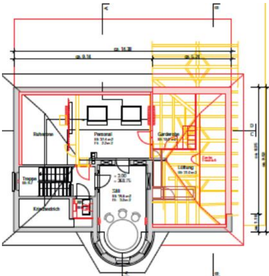
Grundriss Schützenhaus Obergeschoss
