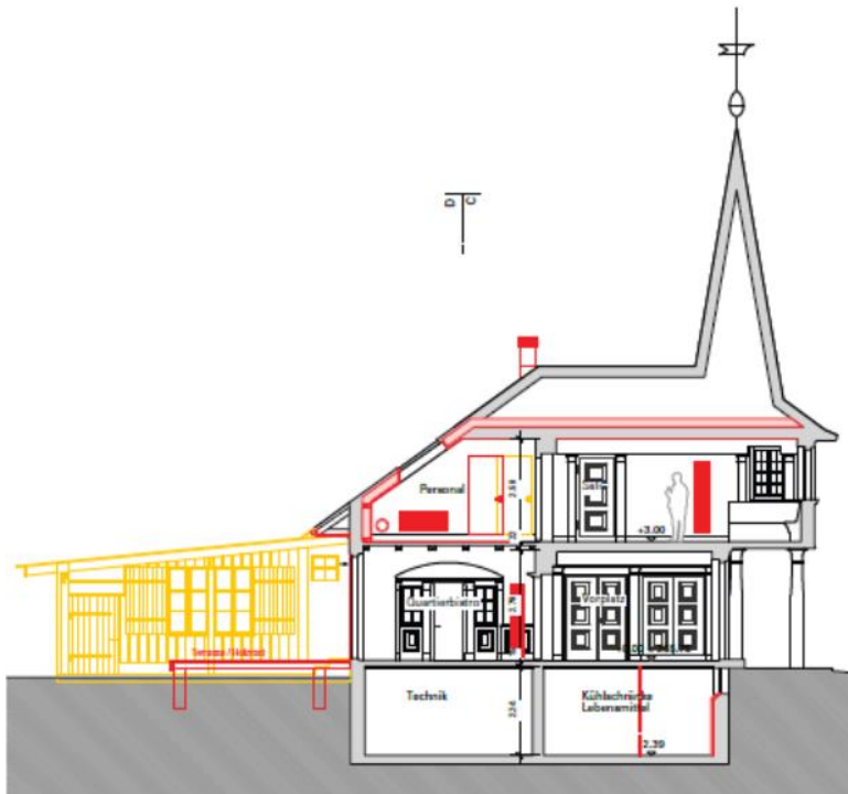
Schnitt AA
