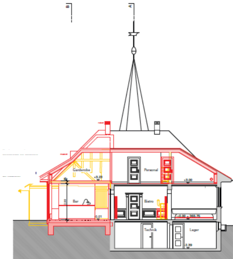
Schnitt CC
