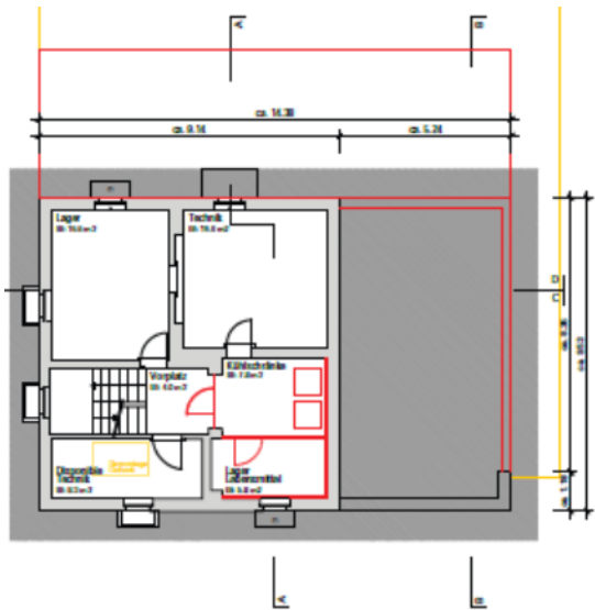
Grundriss Schützenhaus Untergeschoss
