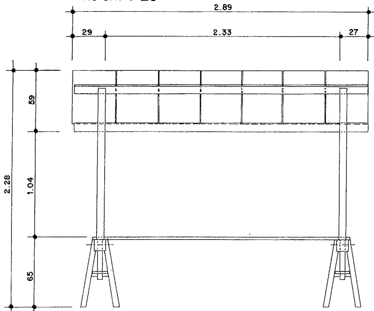
Ansicht 1:25
