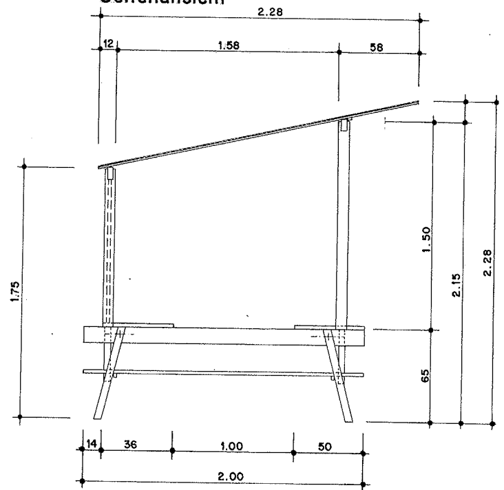
Seitenansicht
