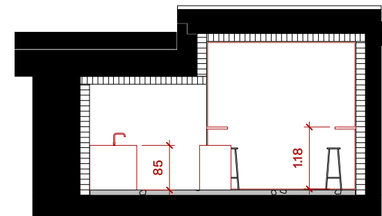
Schnitt B-B
