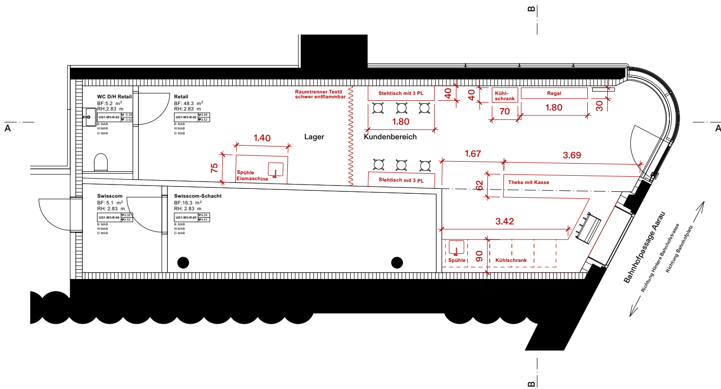
Grundriss Untergeschoss
