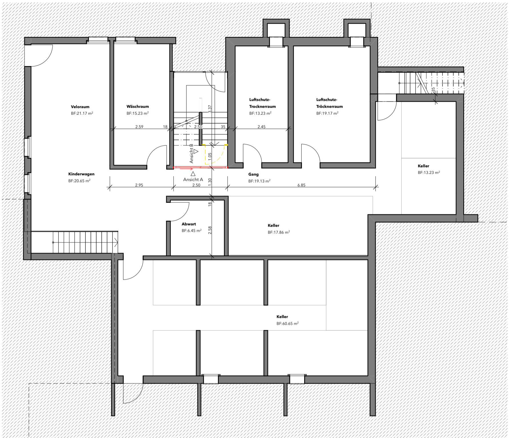
Untergeschoss
