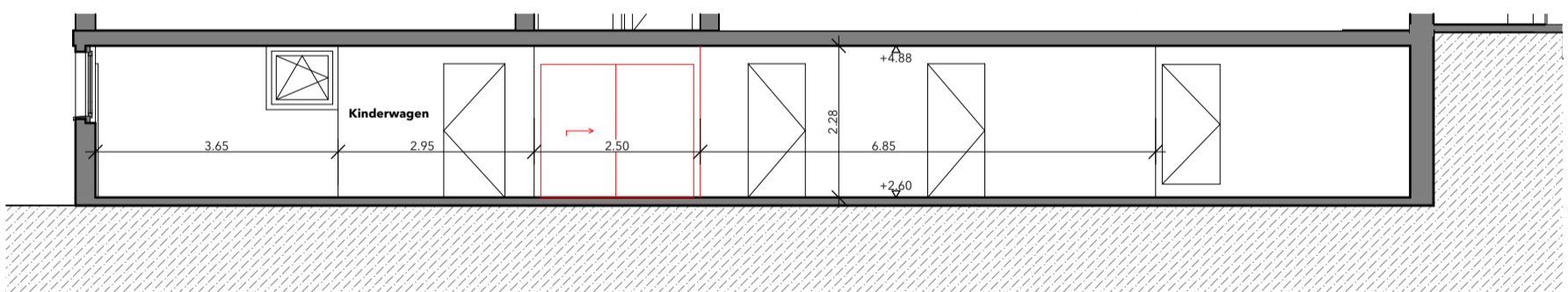
Ansicht A
