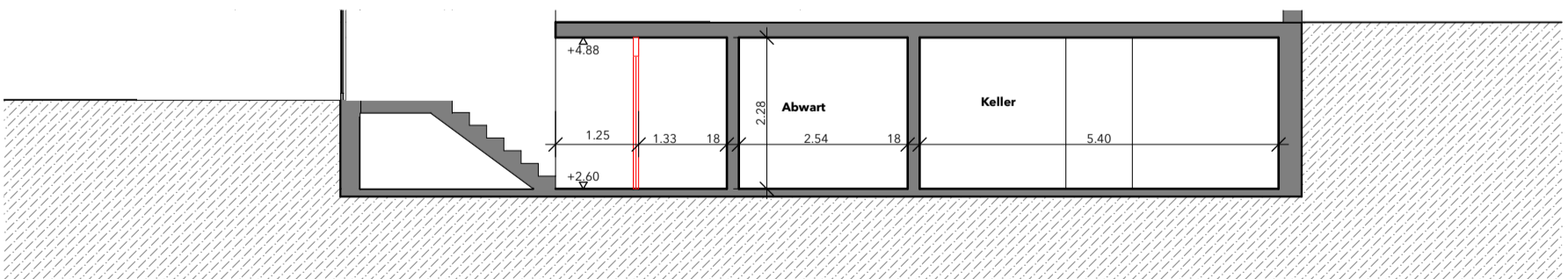
Ansicht B
