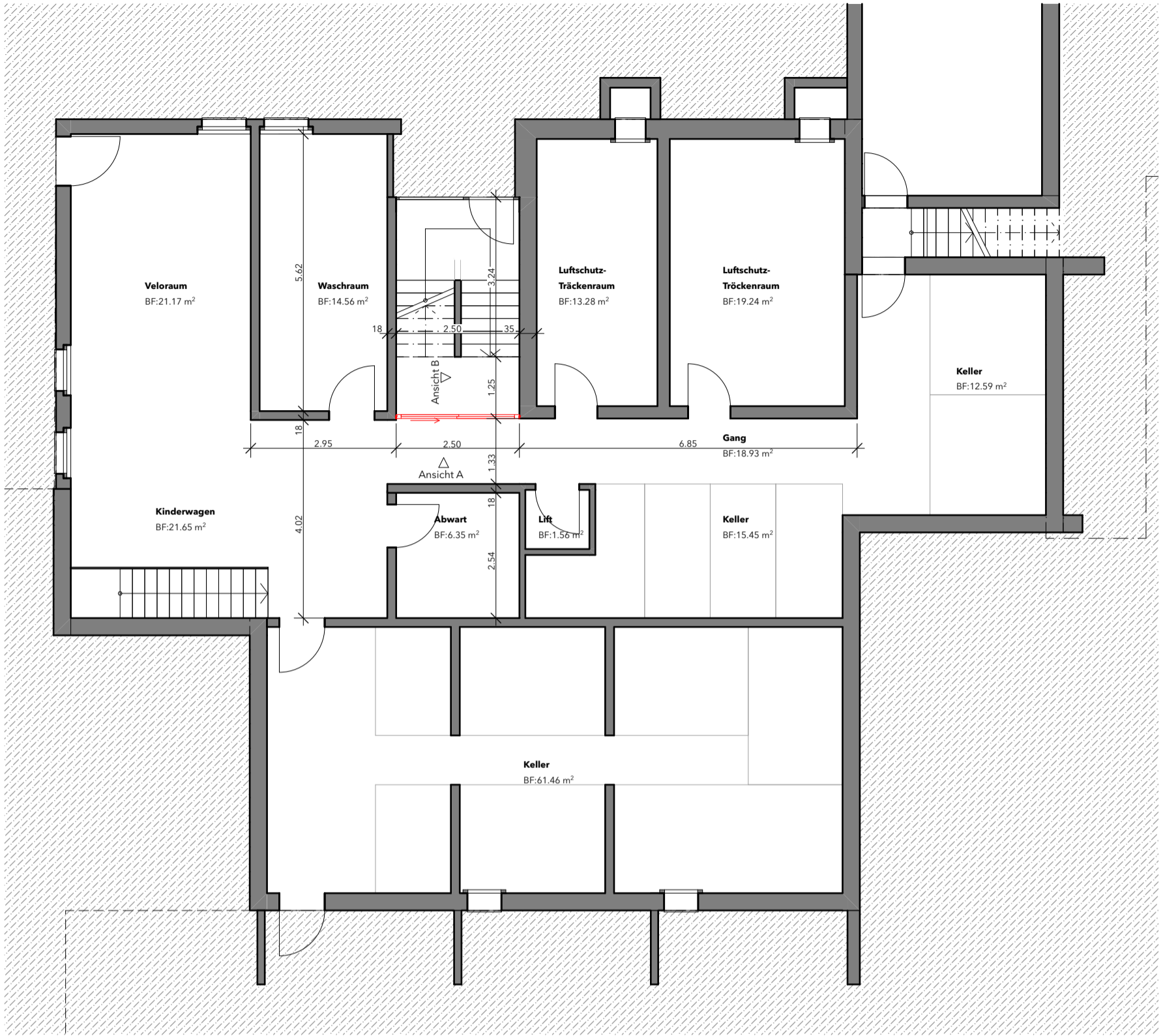
Untergeschoss
