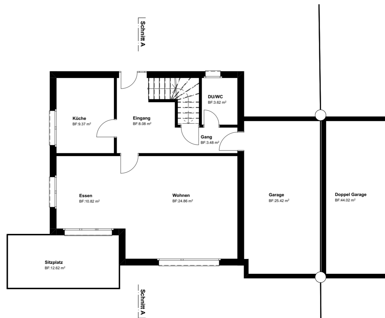
Erdgeschoss
