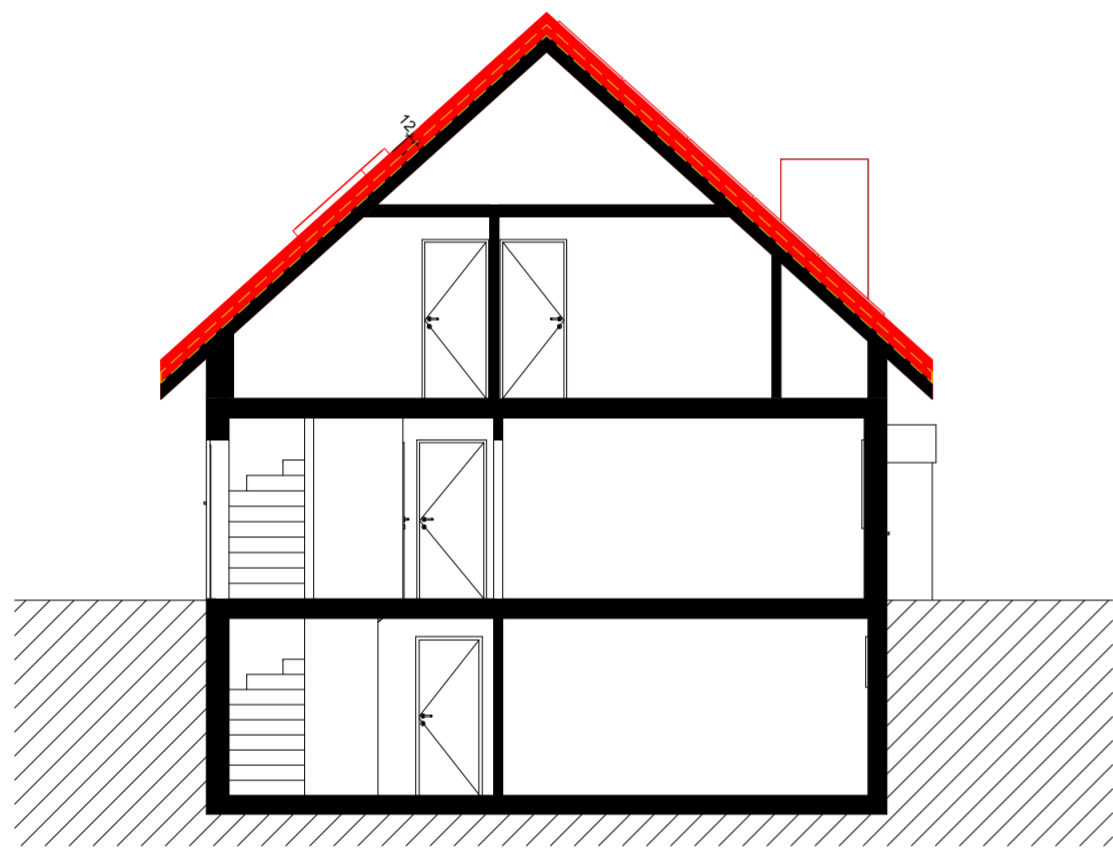
Schnitt A
