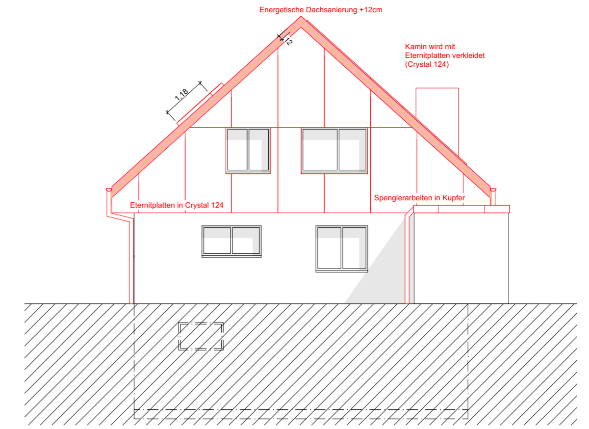
Ansicht Westen
