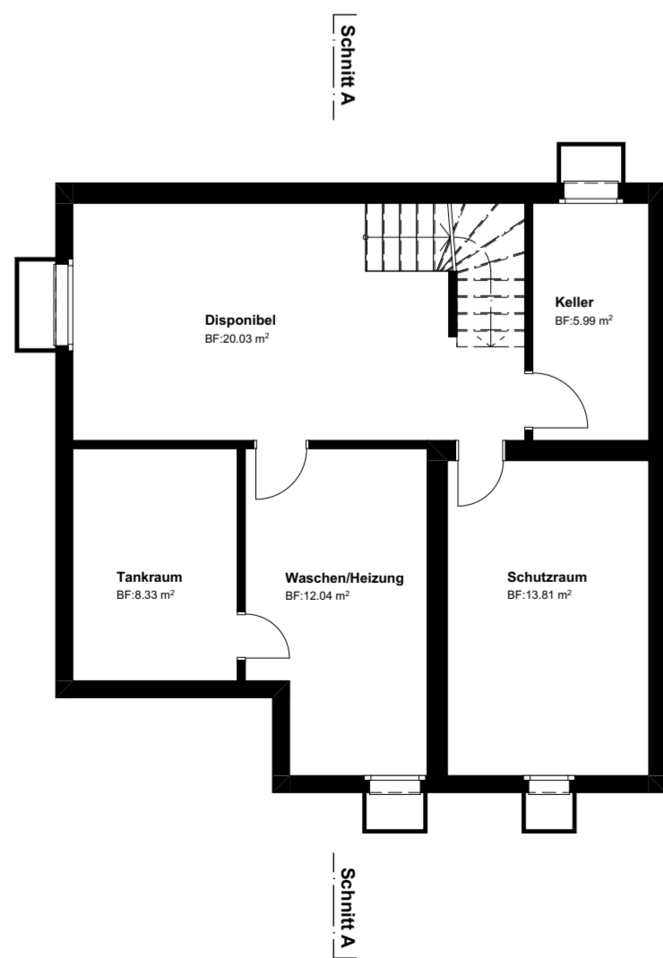
Untergeschoss
