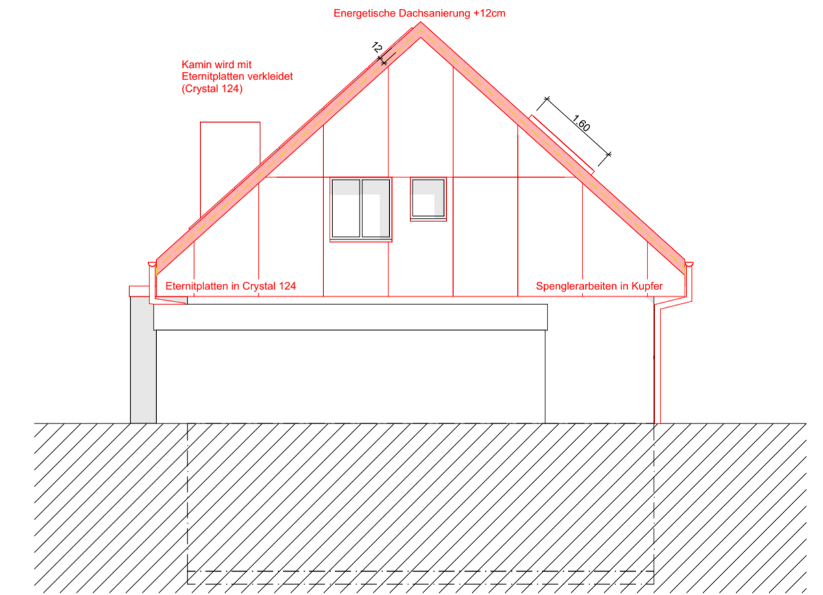
Ansicht Osten
