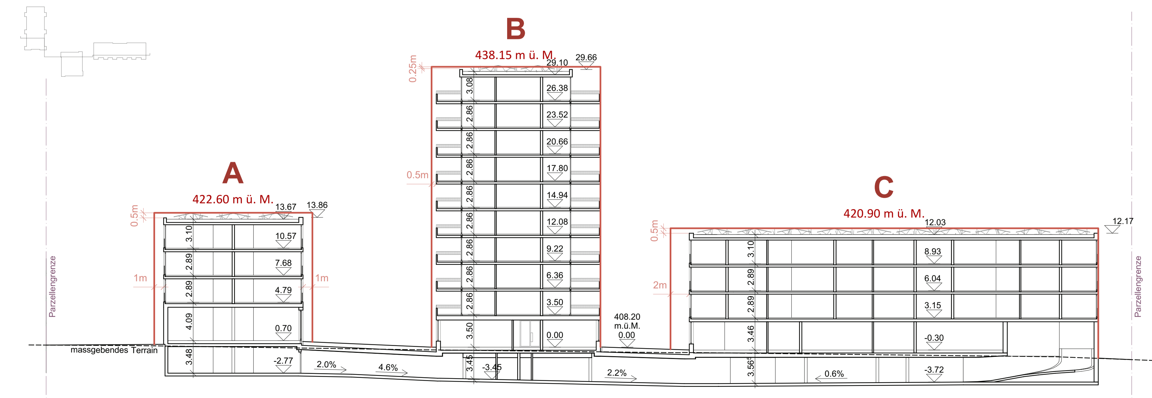
Orientierungsinhalt Schnitt
