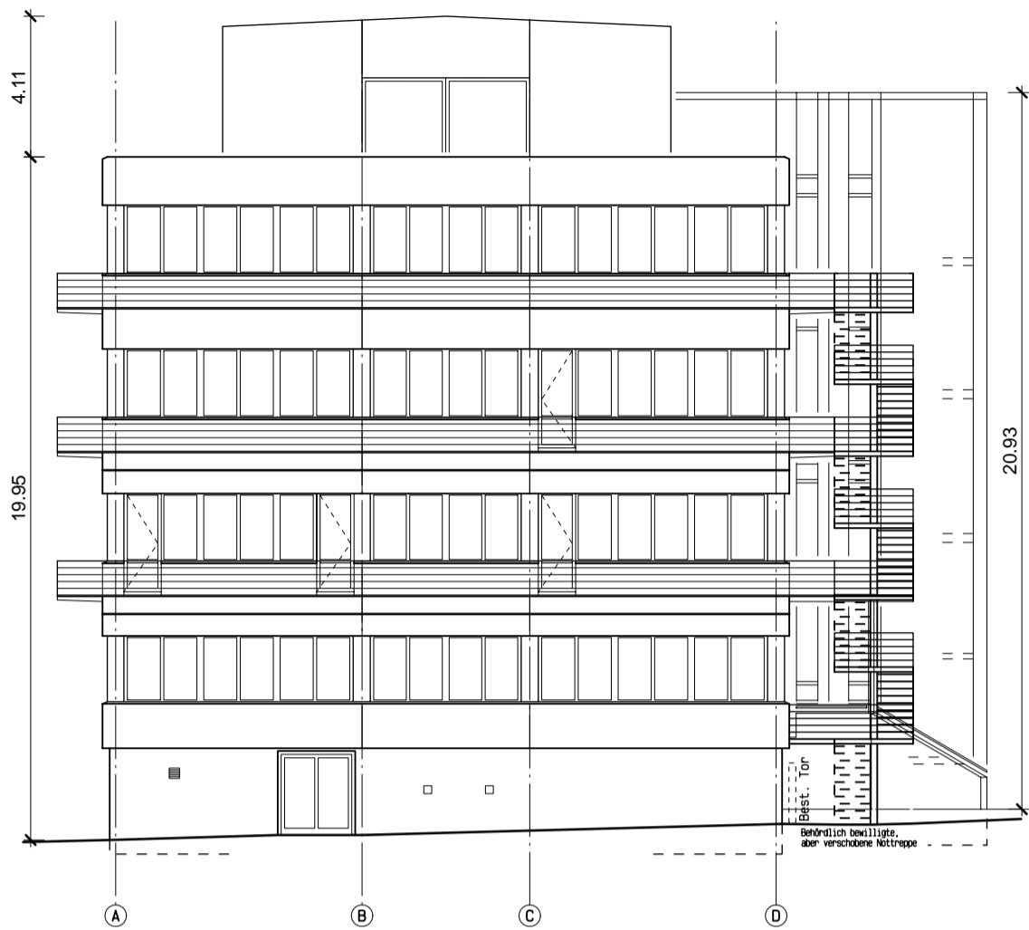
Nordostfassade
