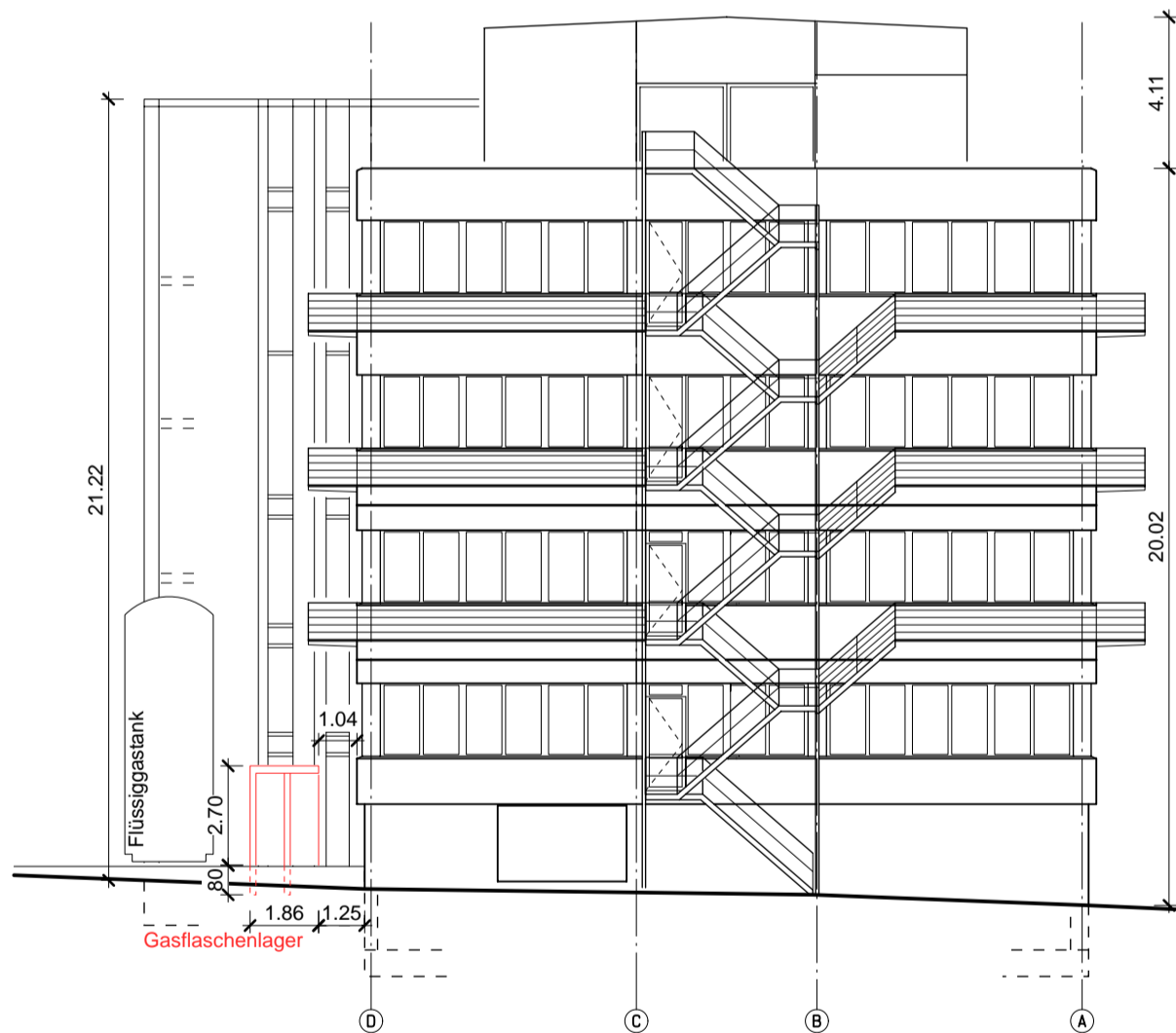
Südwestfassade
