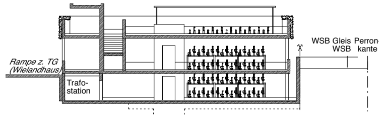
Schnitt C-C
