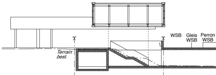
Schnitt B-B
