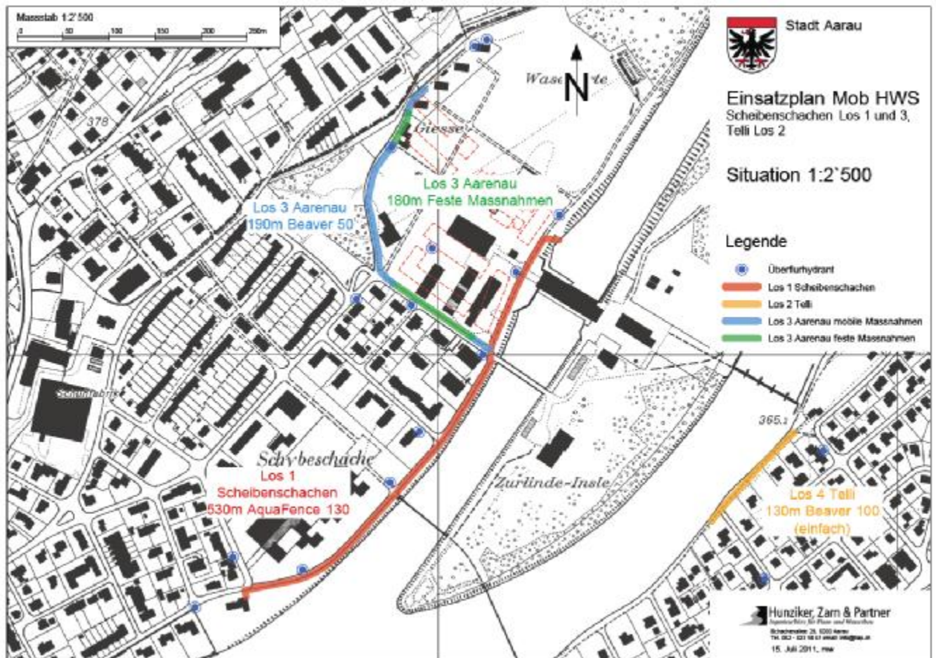
Abbildung 5, Übersichtsplan Hochwasserschutzmassnahmen
