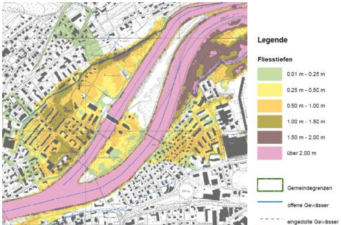
Abbildung 2, Fliesstiefenkarte HQ100
