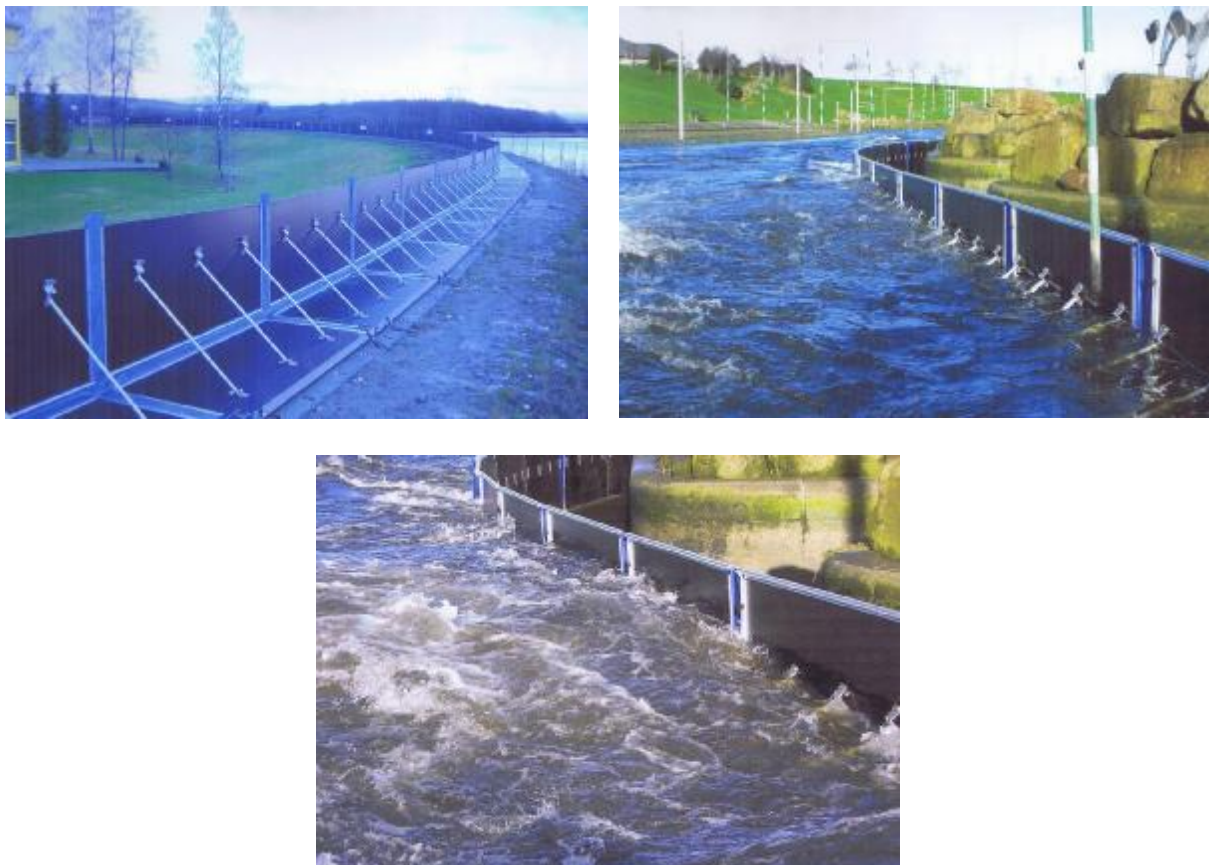
Abbildung 3, Mobile Hochwasserschutz Elemente AquaFence
